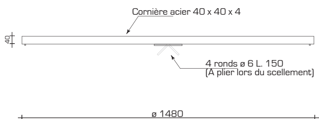
Cadre
