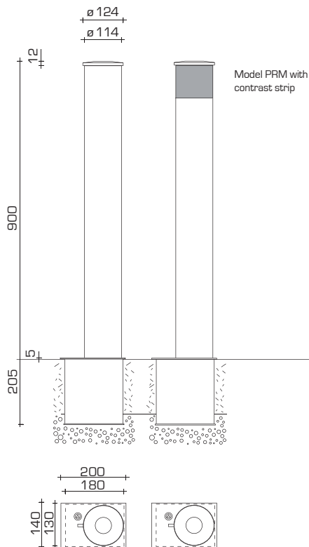
Bollard ø 124
