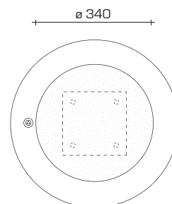
Dessus cendrier
